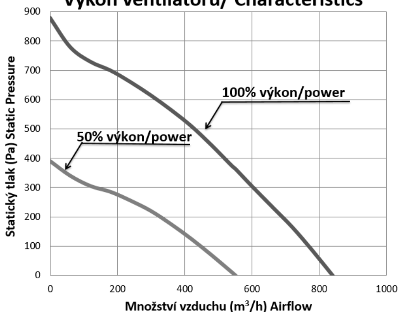
Výkon ventilátoru/ Characteristics
